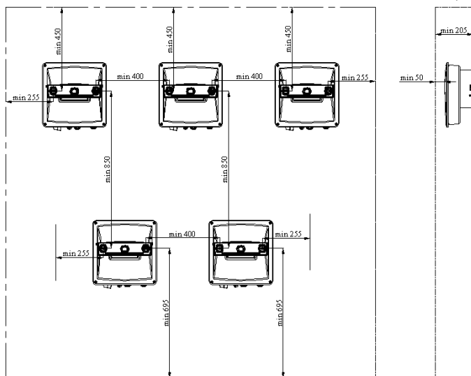
Afstanden bij meerdere omvormers
